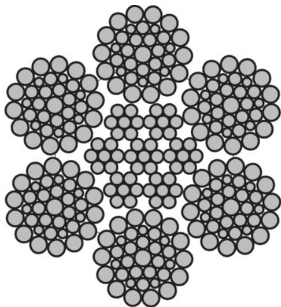
Teräsköysiraksi
